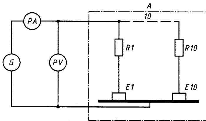
Рисунок 1 — Схема для измерения сопротивления изоляционного покрытия
